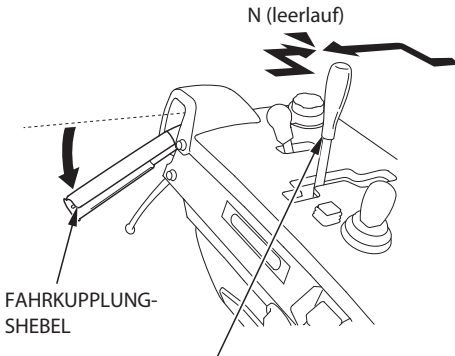
HAUPTGANGSCHALTHEBEL
