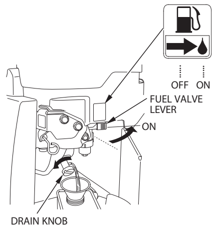
DRAIN KNOB
